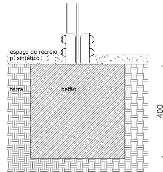
ESQUEMA DE FIXAÇÃO POR SAPATA
