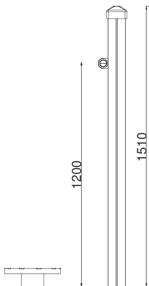
ALÇADO LATERAL
