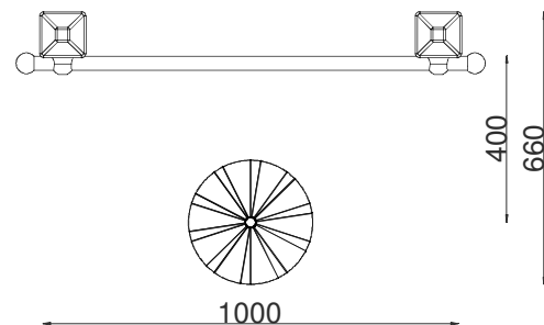
PLANTA
