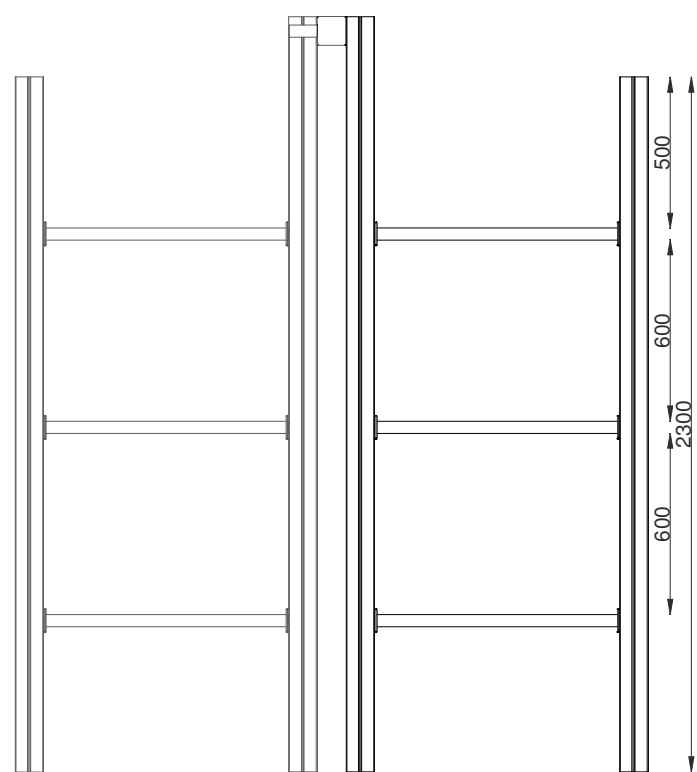
ALÇADO LATERAL
