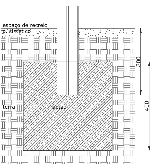
ESQUEMA DE FIXAÇÃO POR ENTERRAMENTO
