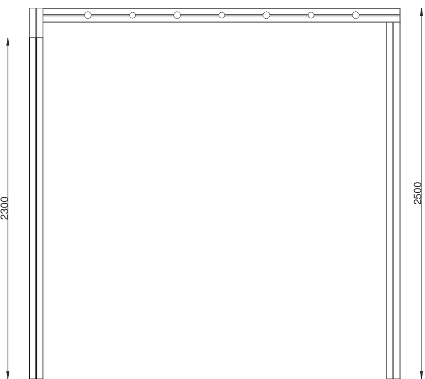
ALÇADO LATERAL
