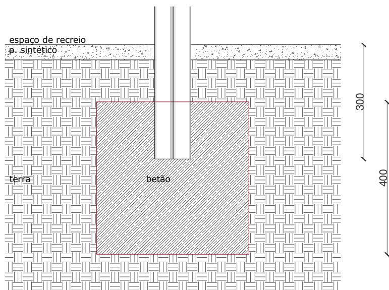
ESQUEMA DE FIXAÇÃO POR ENTERRAMENTO
