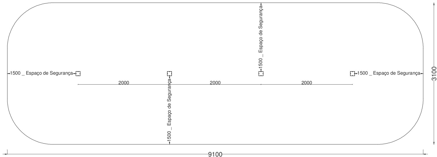
PLANTA - ENQUADRAMENTO DO EQUIPAMENTO NO ESPAÇO DE SEGURANÇA NECESSÁRIO
