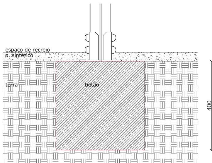
ESQUEMA DE FIXAÇÃO POR SAPATA
