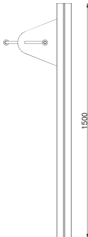
ALÇADO LATERAL
