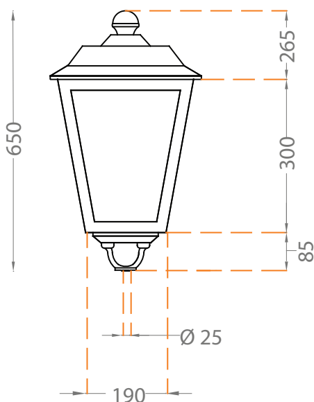
ALÇADO FRONTAL
