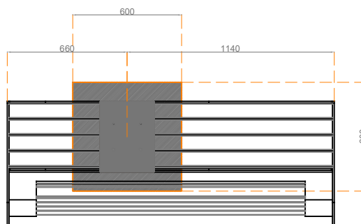
PLANTA . ESQUEMA MACIÇO
