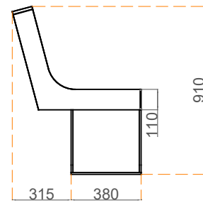
ALÇADO LATERAL
