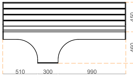
ALÇADO FRONTAL
