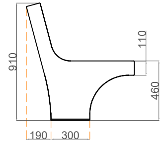
ALÇADO LATERAL
