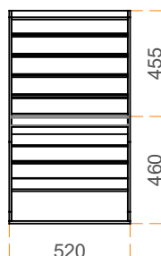
ALÇADO FRONTAL
