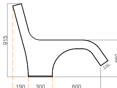
ALÇADO LATERAL
