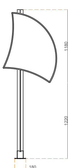
ALÇADO FRONTAL
