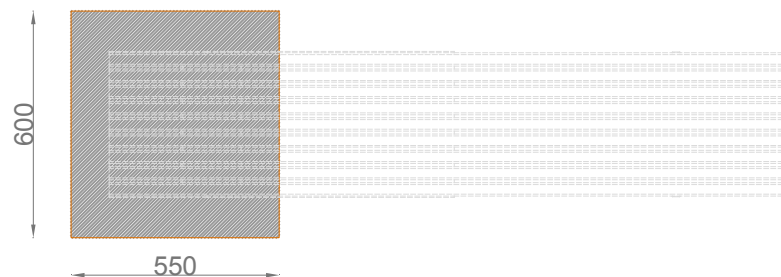
PLANTA . ESQUEMA DE MACIÇOS
