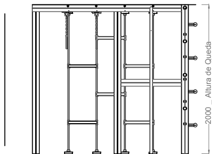
ALÇADO - INDICAÇÃO DA ALTURA DE QUEDA DO EQUIPAMENTO
