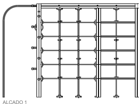
ALÇADO 1
