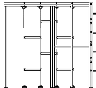
ALÇADO 4
