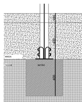
ESQUEMA DE FIXAÇÃO (PISO EM AREIA)
