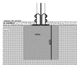
ESQUEMA DE FIXAÇÃO (PISO SINTÉTICO)
