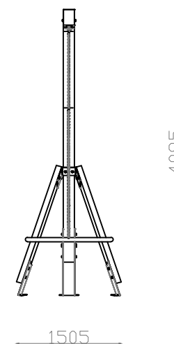
ALÇADO LATERAL
