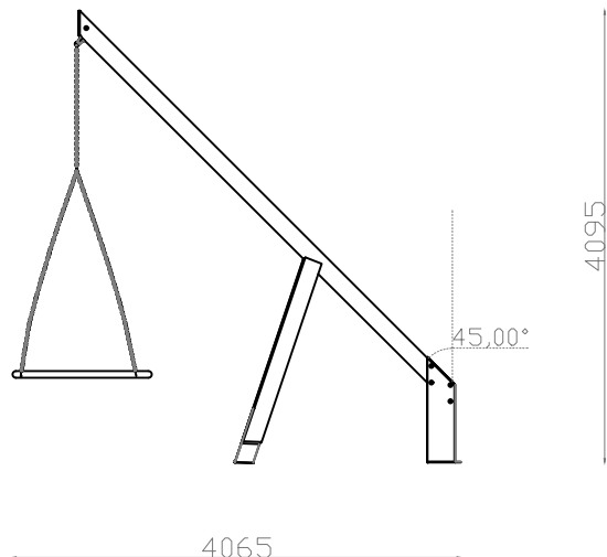
ALÇADO FRONTAL
