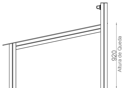
ALÇADO - INDICAÇÃO DA ALTURA DE QUEDA
