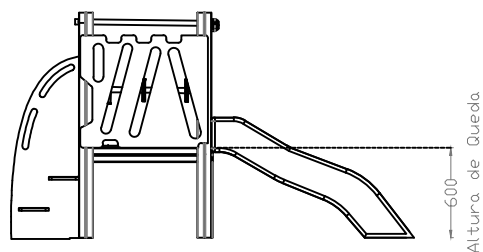
ALÇADO . INDICAÇÃO DE ALTURA DE QUEDA
