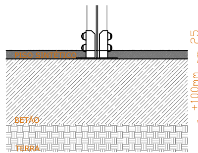
ESQUEMA DE FIXAÇÃO (PISO SINTÉTICO)
