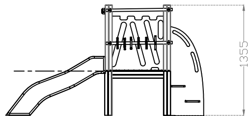
ALÇADO LATERAL DIREITO
