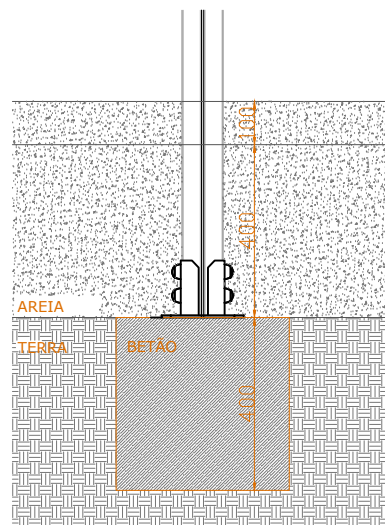
ESQUEMA DE FIXAÇÃO (PISO DE AREIA)
