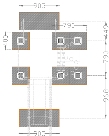
PLANTA . ESQUEMA DE MACIÇOS
