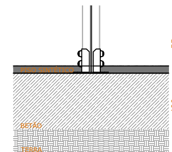
ESQUEMA DE FIXAÇÃO (PISO SINTÉTICO)
