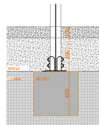
ESQUEMA DE FIXAÇÃO (PISO DE AREIA)
