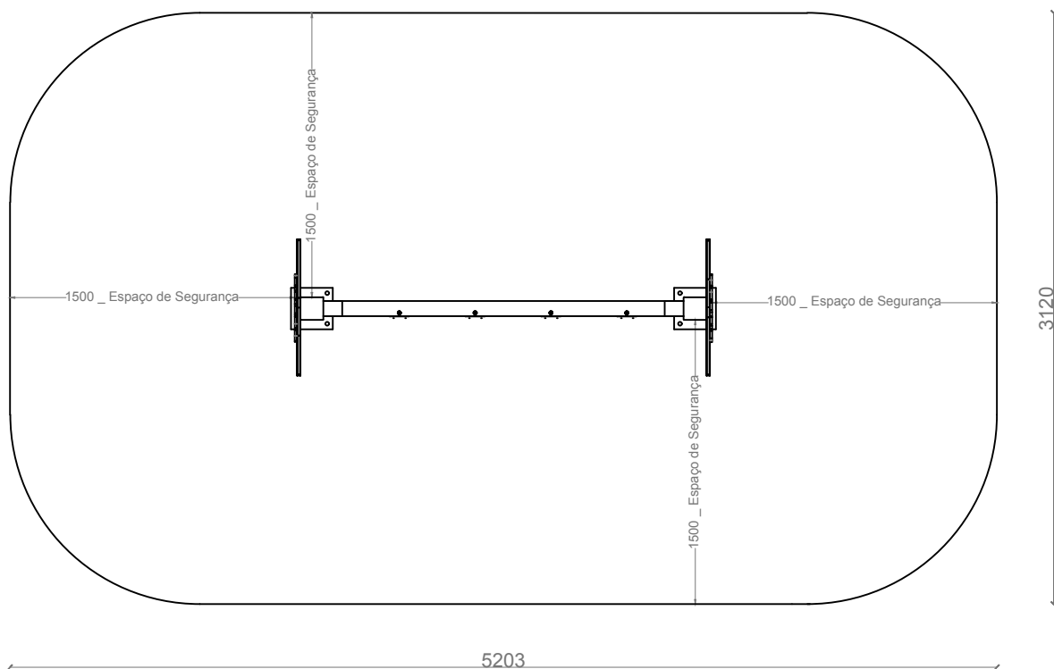
PLANTA - ENQUADRAMENTO DO EQUIPAMENTO NO ESPAÇO DE SEGURANÇA NECESSÁRIO
