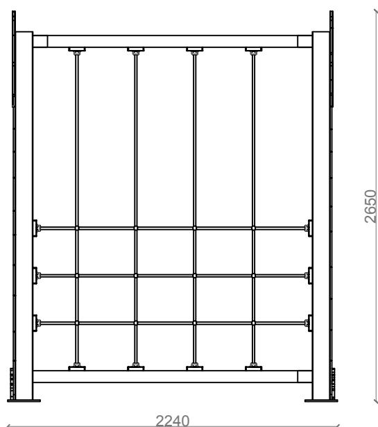
ALÇADO FRONTAL
