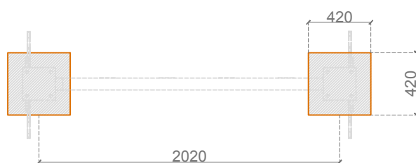
MACIÇOS DE BETÃO dimensões _ 420x420x400mm
