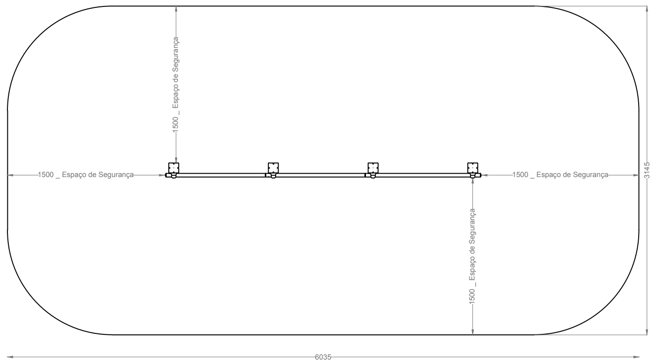
PLANTA - ENQUADRAMENTO DO EQUIPAMENTO NO ESPAÇO DE SEGURANÇA NECESSÁRIO
