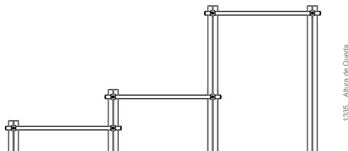
ALÇADO - INDICAÇÃO DA ALTURA DE QUEDA
