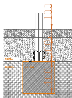
ESQUEMA DE FIXAÇÃO (PISO DE AREIA)
