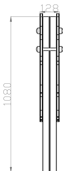
Vista lateral
