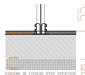
ESQUEMA DE FIXAÇÃO (PISO SINTÉTICO)
