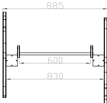
Planta
