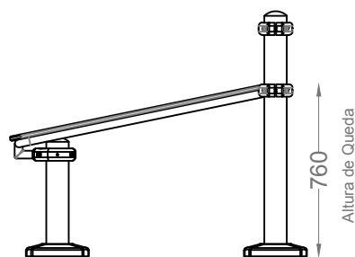
ALÇADO - INDICAÇÃO DA ALTURA DE QUEDA
