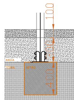
ESQUEMA DE FIXAÇÃO (PISO DE AREIA)
