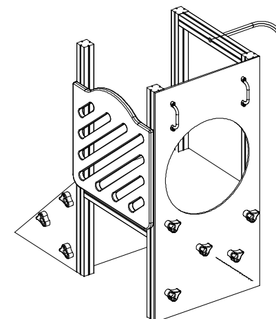
VISTA AXONOMÉTRICA DO EQUIPAMENTO
