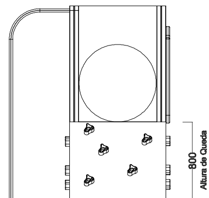
ALÇADO - INDICAÇÃO DA ALTURA DE QUEDA DO EQUIPAMENTO
