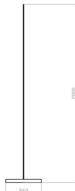
VISTA LATERAL
