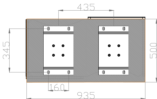
PLANTA - ESQUEMA DE MACIÇOS
