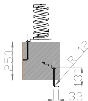
ALÇADO . Esquema de Fixação
