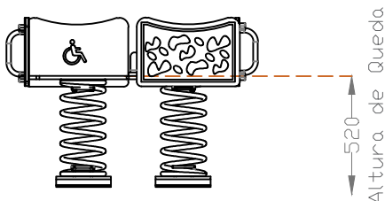
ALÇADO - INDICAÇÃO DA ALTURA DE QUEDA DO EQUIPAMENTO
