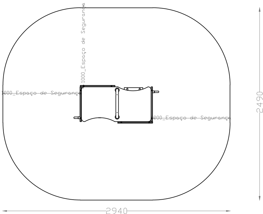
PLANTA - ENQUADRAMENTO DO EQUIPAMENTO NO ESPAÇO DE SEGURANÇA NECESSÁRIO
