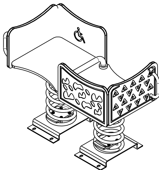
Vista Isométrica
