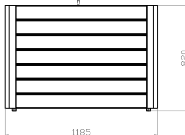
ALÇADO LATERAL
