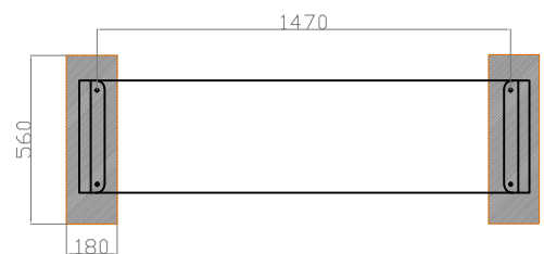
PLANTA - ESQUEMA DE MACIÇOS
