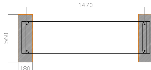
PLANTA - ESQUEMA DE MACIÇOS
