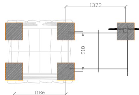
ESQUEMA DE MACIÇOS DIMENSÕES: 400 x 400 x 400 mm
