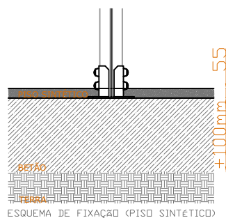
ESQUEMA DE FIXAÇÃO (PISO SINTÉTICO)
