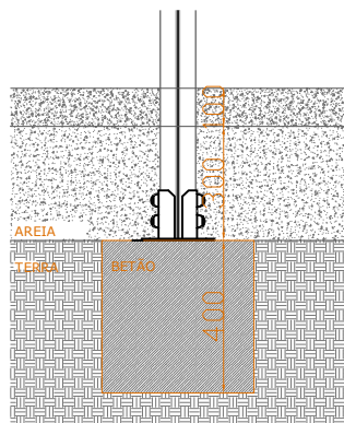
ESQUEMA DE FIXAÇÃO (PISO DE AREIA)
