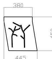
ALÇADO LATERAL
