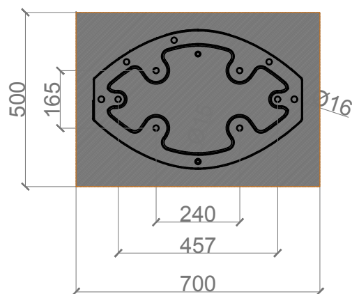
PLANTA - ESQUEMA DE MACIÇOS
