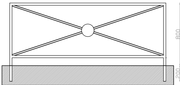
ALÇADO FRONTAL
