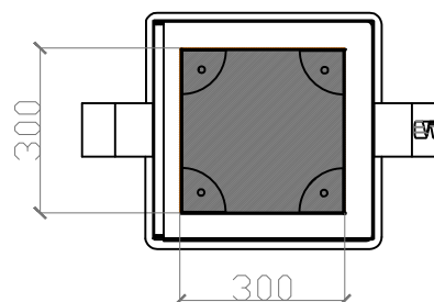
PLANTA - ESQUEMA DE MACIÇOS
