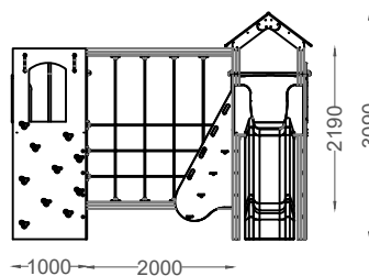
ALÇADO FRONTAL FRONT VIEW
