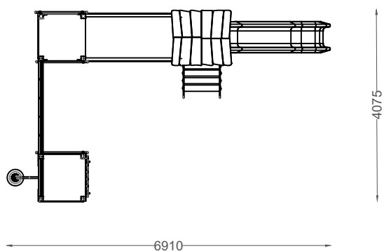
PLANTA PLAN
