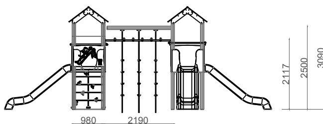
ALÇADO FRONTAL FRONT VIEW
