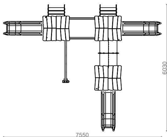
PLANTA PLAN
