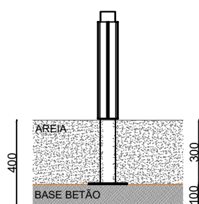
PLANTA . ESQUEMA DE FIXAÇÃO PLAN . INSTALLATION PLAN
