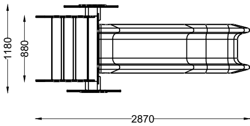
PLANTA PLAN
