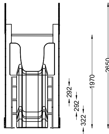
ALÇADO FRONTAL FRONT VIEW
