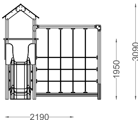
ALÇADO FRONTAL FRONT VIEW
