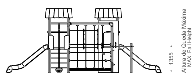
ALÇADO FRONTAL FRONT VIEW
