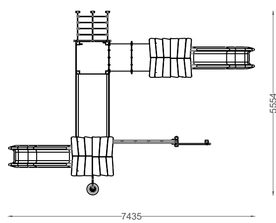
PLANTA PLAN
