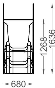
ALÇADO FRONTAL FRONT VIEW
