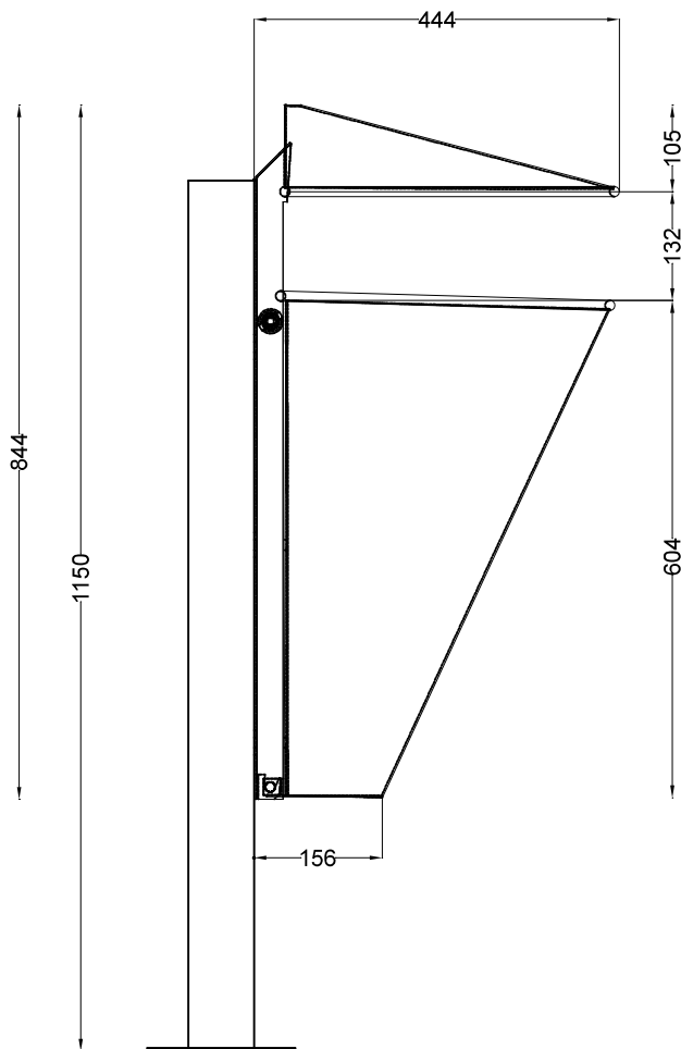
ALÇADO LATERAL
