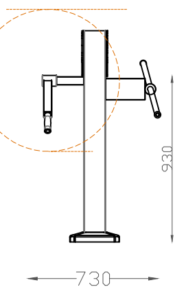
ALÇADO LATERAL SIDE VIEW
