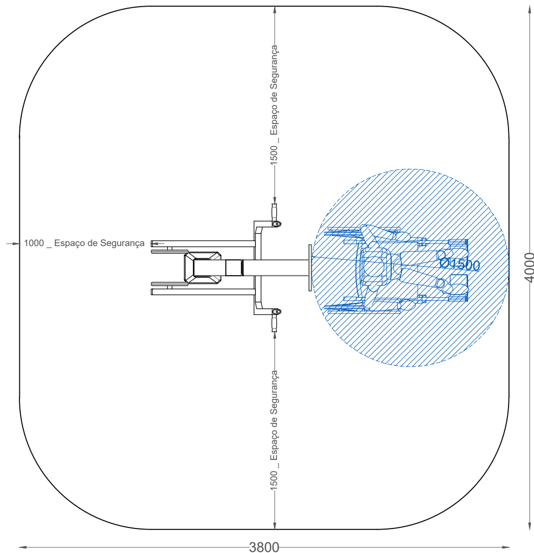
PLANTA - ESPAÇO DE SEGURANÇA NECESSÁRIO PLAN - SAFETY SPACE REQUIRED
