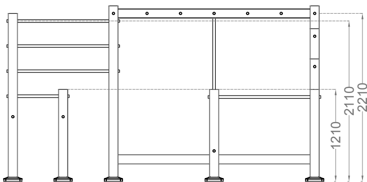
ALÇADO FRONTAL
