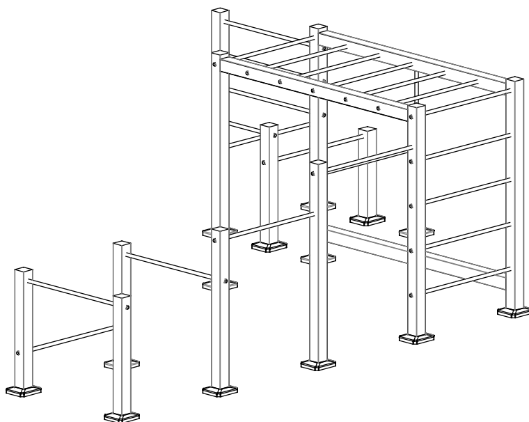
VISTA AXONOMÉTRICA
