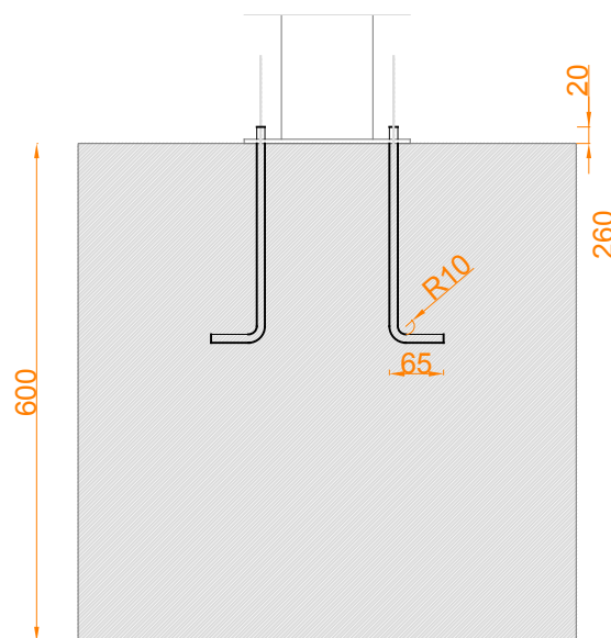
ALÇADO
