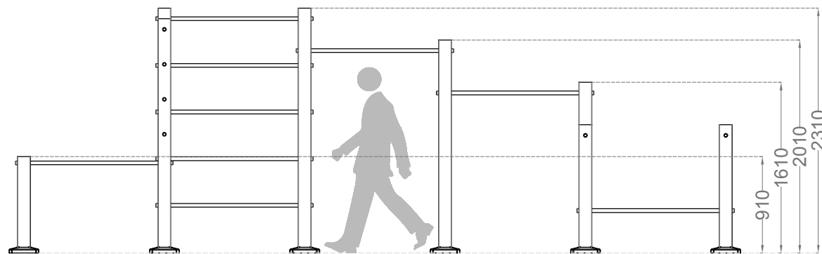
ALÇADO LATERAL
