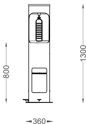
ALÇADO FRONTAL FRONT VIEW
