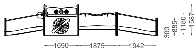
ALÇADO FRONTAL FRONT VIEW
