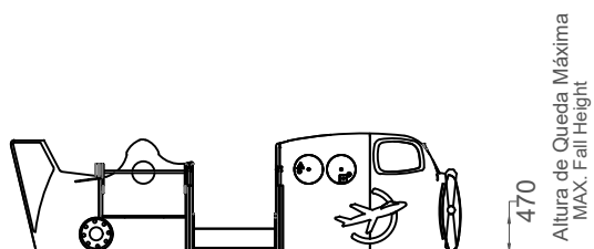
ALÇADO LATERAL SIDE VIEW
