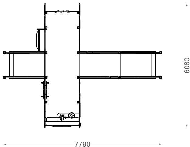
PLANTA PLAN
