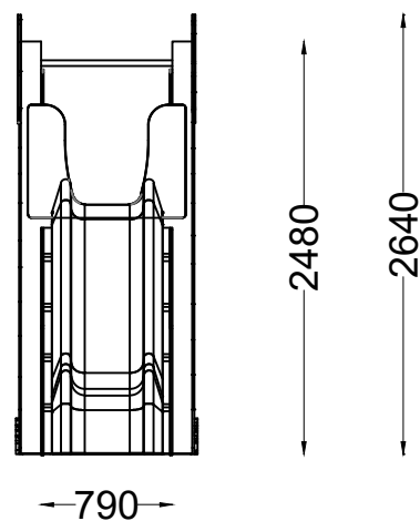
ALÇADO FRONTAL FRONT VIEW
