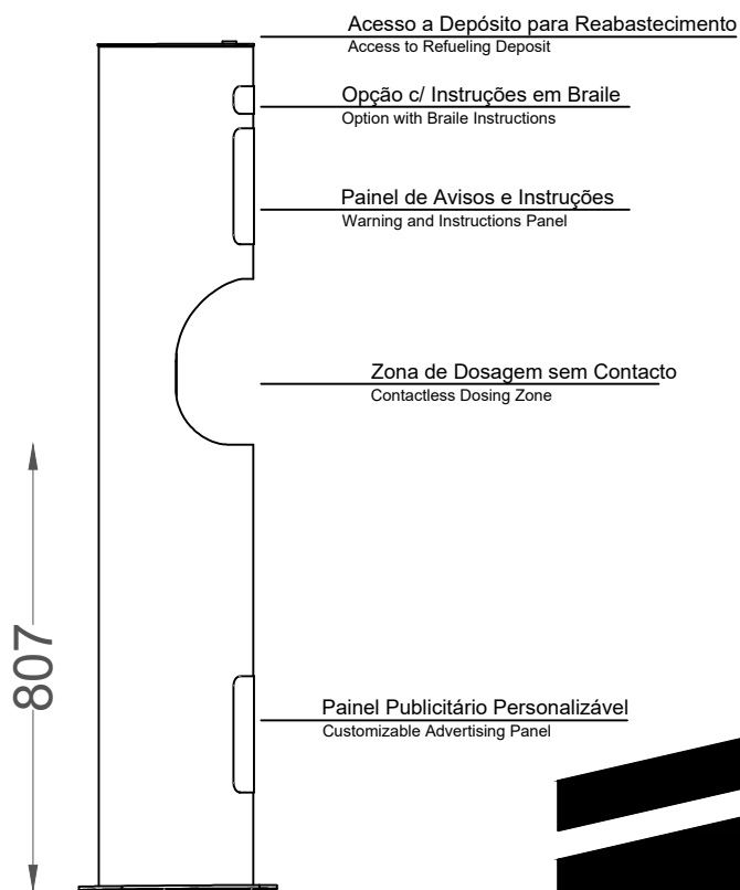
ALÇADO FRONTAL FRONT VIEW
