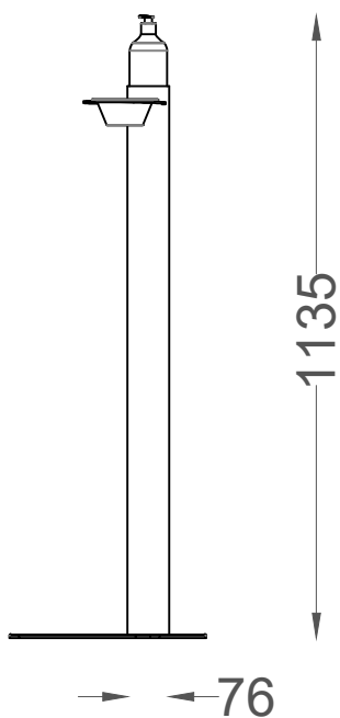
ALÇADO LATERAL SIDE VIEW
