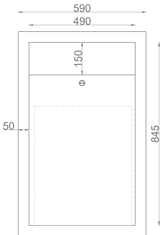
ALÇADO FRONTAL
